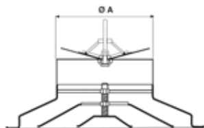
Diffusore con serr. a farfalla
