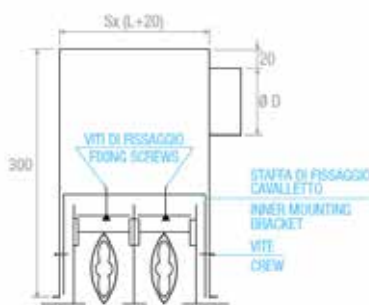
Fissaggio al plenum con staffe CVL cavalletti
