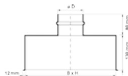
Attacco Verticale (V)
