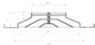
Diffus. 600x600 con serr. a farfalla
