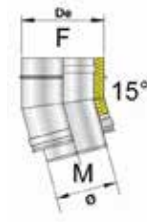
Doppia Parete isol 25mm Int Inox AISI 316L Est Inox AISI 304
