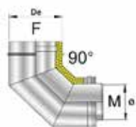
Doppia Parete isol 25mm Int Inox AISI 316L Est Inox AISI 304
