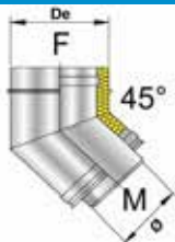
Doppia Parete isol 25mm Int Inox AISI 316L Est Inox AISI 304
