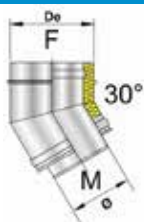
Doppia Parete isol 25mm Int Inox AISI 316L Est Inox AISI 304
